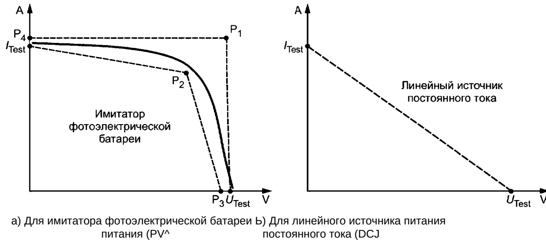
Рисунок 1 — Вольт-амперные характеристики
