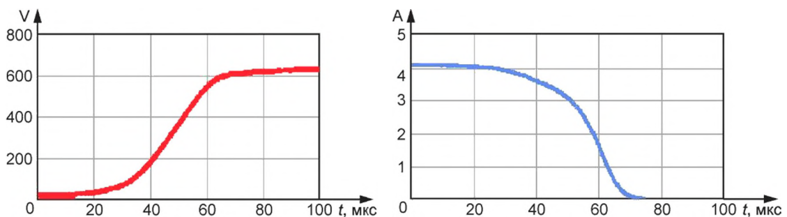
Рисунок В.2 — Характер изменения напряжения и тока во времени в течение рабочего времени отключения полупроводникового переключателя при I_{\text{sc}} имитатора фотоэлектрической батареи, равном 4 А, и напряжении холостого хода, равном 640 В
