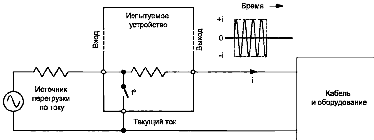
Рисунок В.3 — Параллельный тепловой трехполюсный ограничитель тока (тепловой предохранитель)
