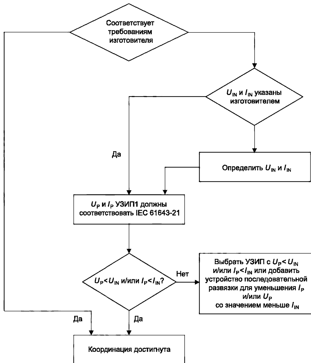
Рисунок Е.1 — Процесс проверки координации
