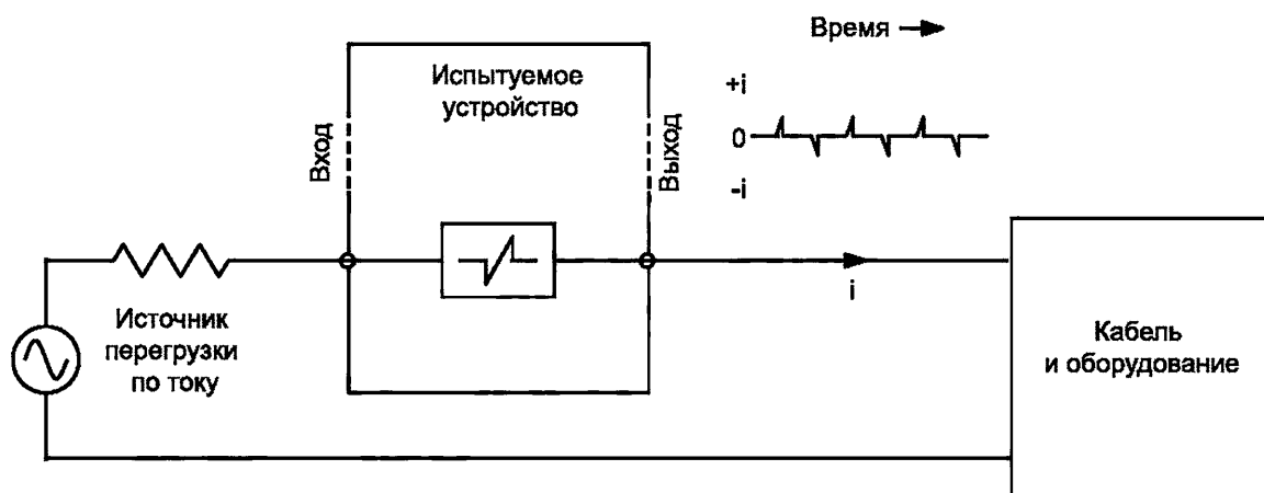
Рисунок В.6 —Двухполюсный последовательный электронный ограничитель тока
