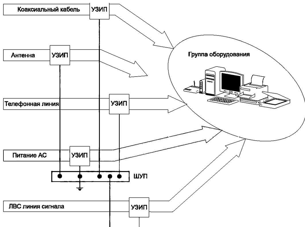
Рисунок 10 — Отдельные УЗИП
