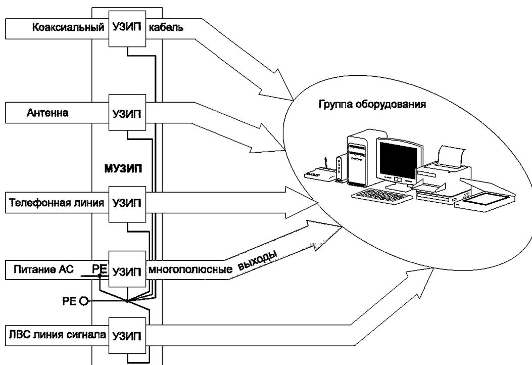
Рисунок 11 — МУЗИП с вариантом подключения к точке заземления (РЕ)
