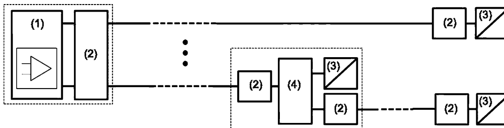
Рисунок 1 — Монтаж УЗИП в сетях телекоммуникаций и сигнализации
