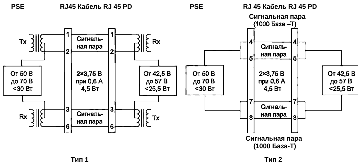
Рисунок F.1 — Режимы питания PoE
