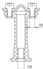
СЕЧЕНИЕ А-А
