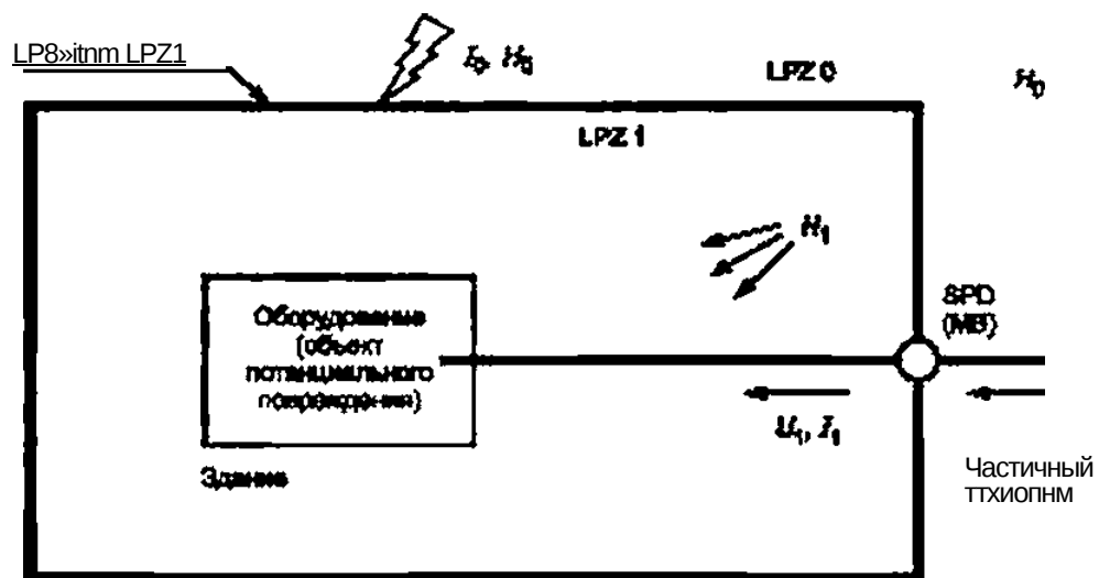
Рисунок 2б — Применение пространственного экрана и устройства защиты SPD на входе в зону LPZ в качестве меры защиты SPM. Оборудование защищено от перенапряжений, передаваемых проводным путем ( I_1 < I_{sp} и I_1 < I_0 ) и от наведенных магнитных полей ( H_1 < H_0 )
