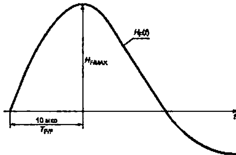
Рисунок А.2в — Моделирование нарастания магнитного поля первого положительного удара молнии (10/350 мкс) при помощи одиночного импульса 8/20 мкс (затухающее колебание 25 кГц)
