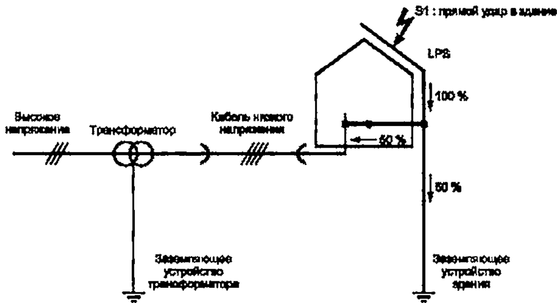
Рисунок 0.3 — Характерный пример сбалансированного распределения тока
