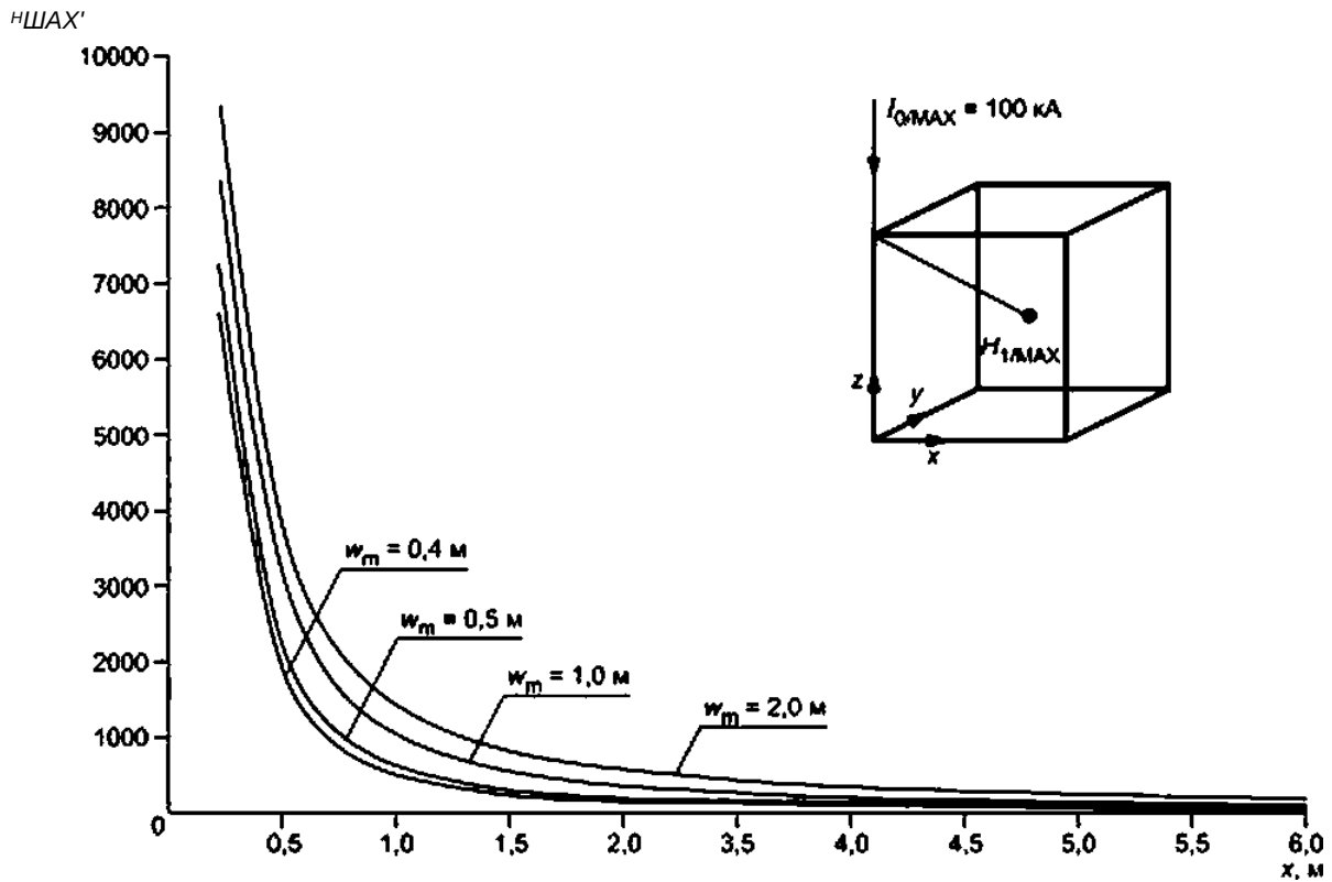
Рисунок А. 11 — Напряженность магнитного поля
