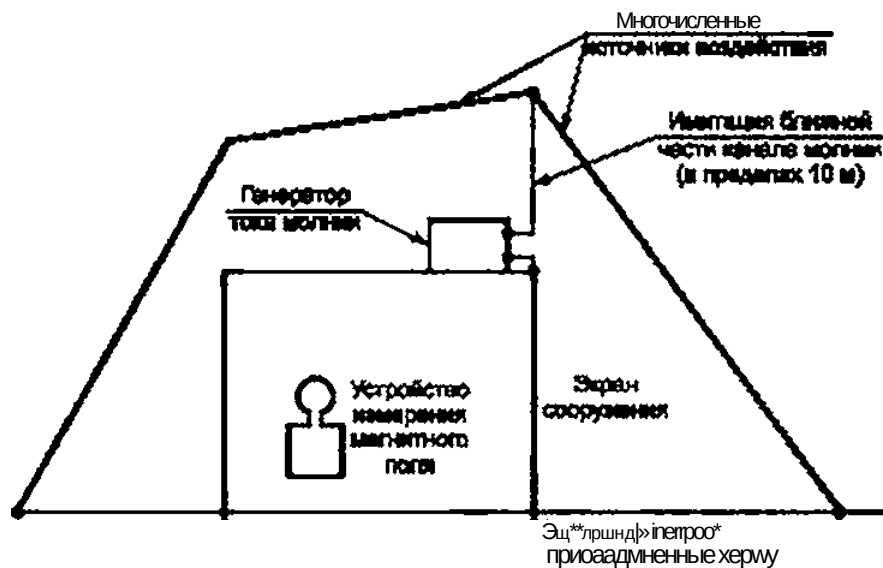
Рисунок А. 13а — Испытательная установка
