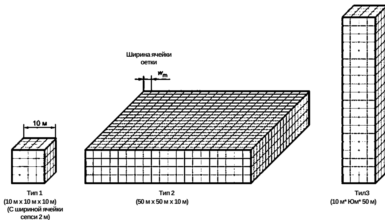
Рисунок А.10 — Типы экранов большого объема, выполненных в виде сетки
