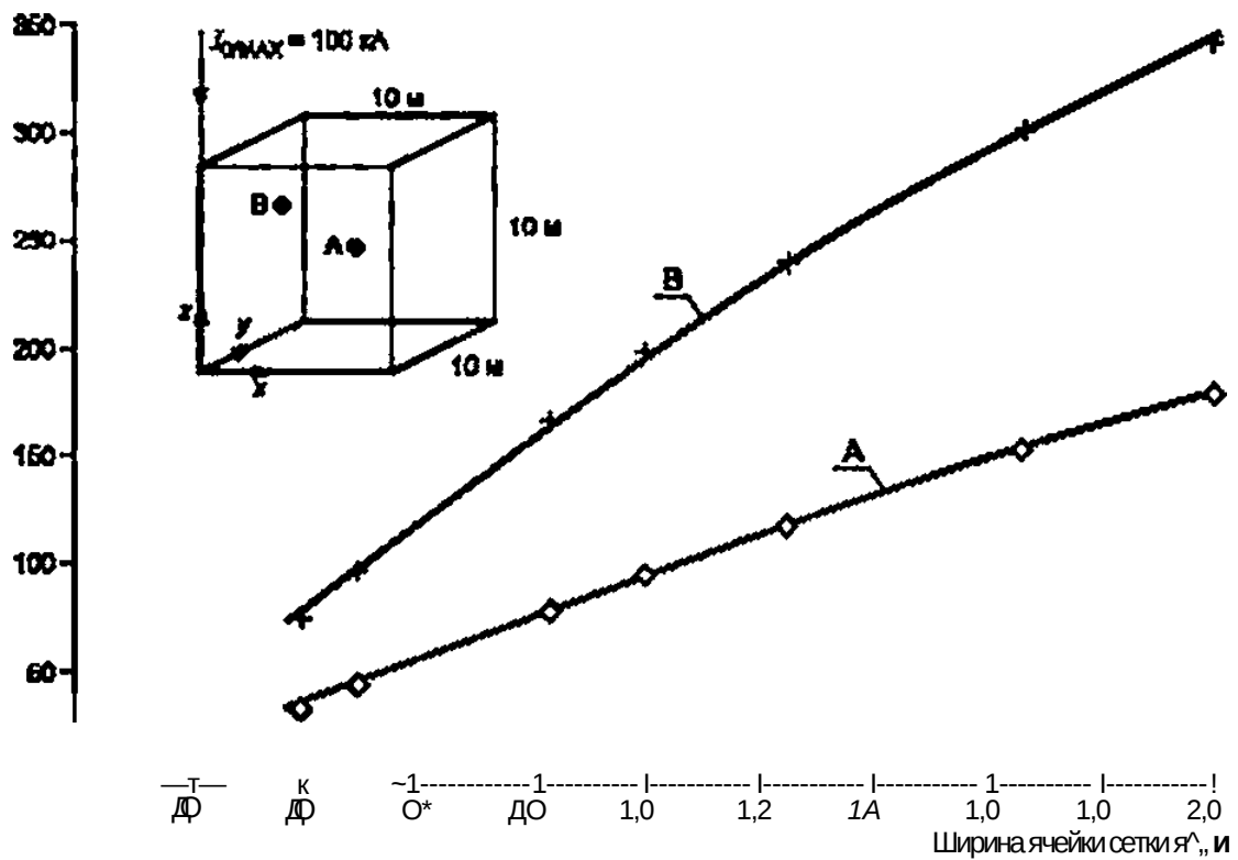
Рисунок А. 12 — Напряженность магнитного поля H_{1/Ax} внутри экрана типа 1 в зависимости от ширины ячейки сетки
