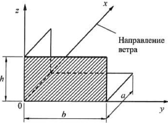
Рисунок 11.2 - Основная система координат при определении коэффициента корреляции \psi
