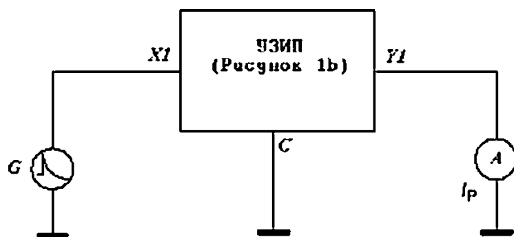
Рисунок Е.2 - Определение сквозного тока общего вида
