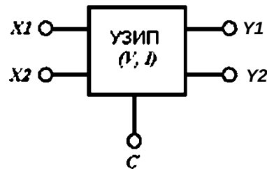
10 - четырехвыводное УЗИП
