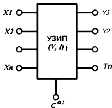
1е - пятивыводное УЗИП
