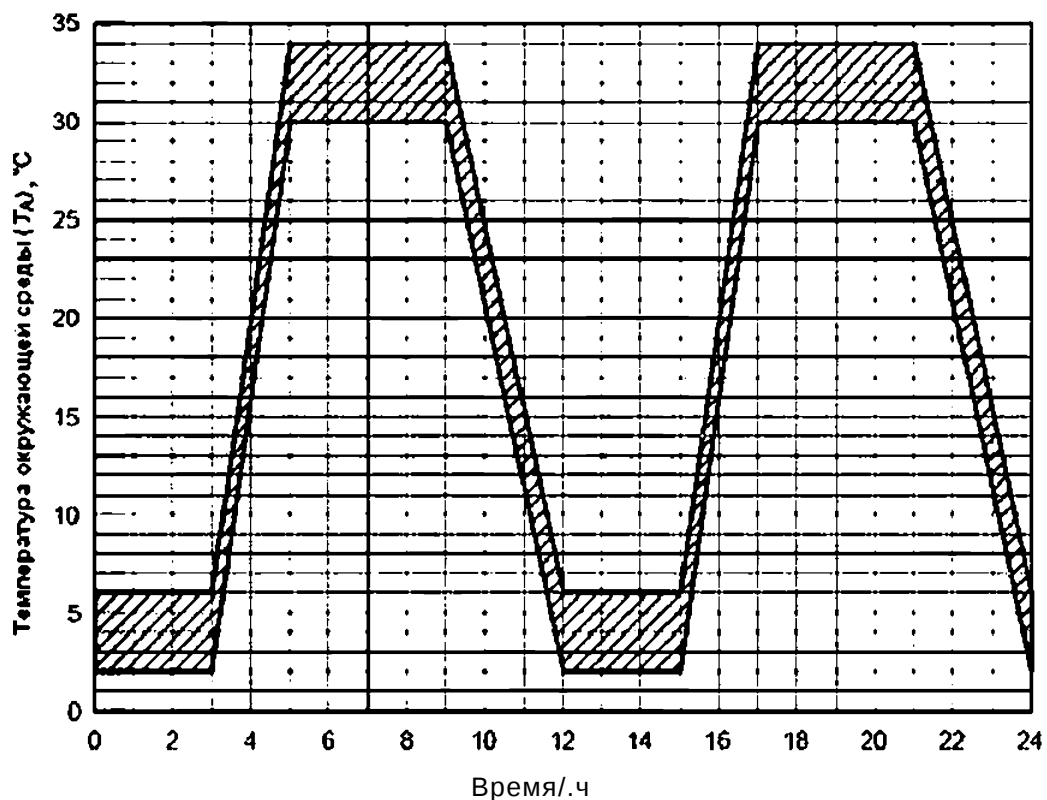
Рисунок 14 - Шкала А циклического воздействия окружающей среды при относительной влажности \Phi 90%
