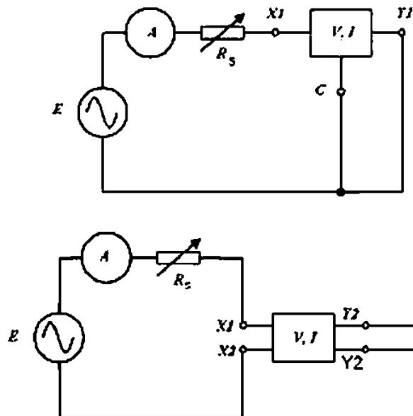
Рисунок 5 - Испытательные цепи для проверки номинального тока, последовательного сопротивления, времени срабатывания, времени возврата тока, максимального напряжения отключения и рабочего режима
