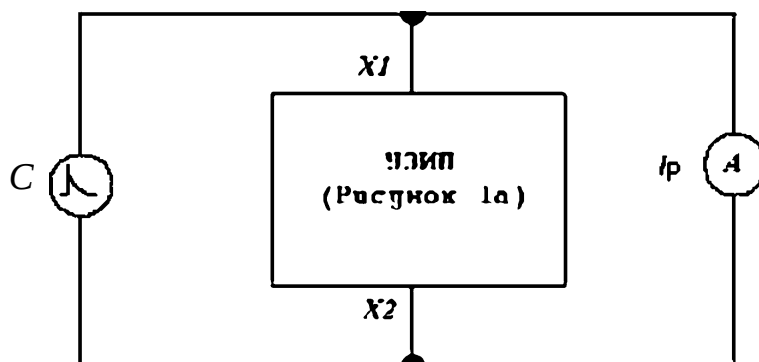
Рисунок Е.1 - Определение сквозного тока дифференциального вида
