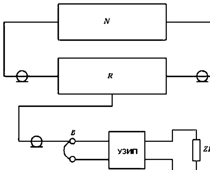
Рисунок 8 - Испытательные цепи для проверки потерь при вводе
