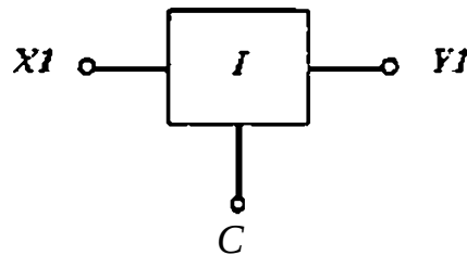
А.1б - Трехвыводной токоограничитель
