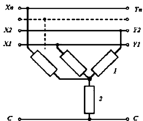
Цель защиты, соединенная звездой
