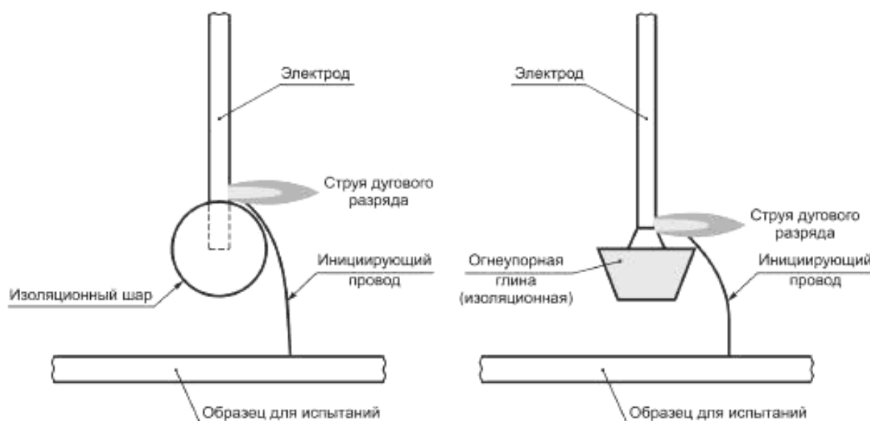
Рисунок D.10 — Стандартные испытательные электроды с отведением струи
