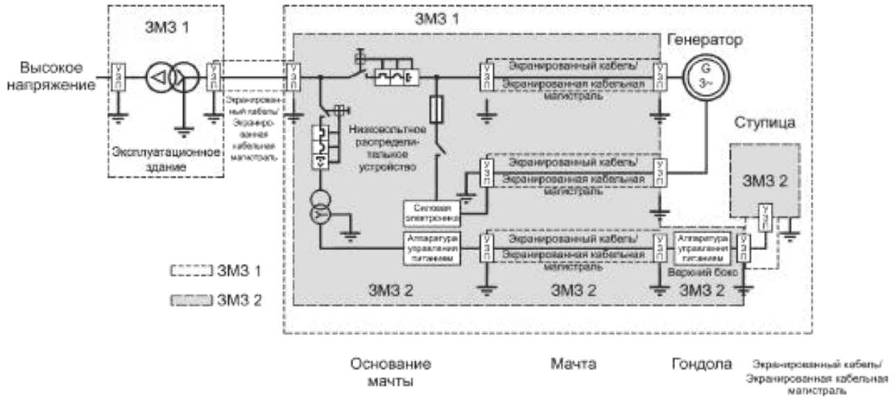
Рисунок Е.6 — Пример записи деления мер защиты электрической системы от электромагнитного импульса от грозовых разрядов на зоны защиты с указанием мест пересечения с электрической целью границ ЗМЗ, показывающий как длинные кабели проходят между основанием мачты и гондолой
