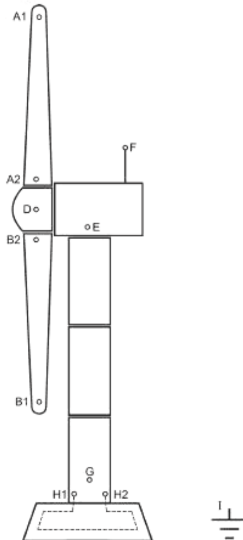
Рисунок J.1 — Пример точек измерения
