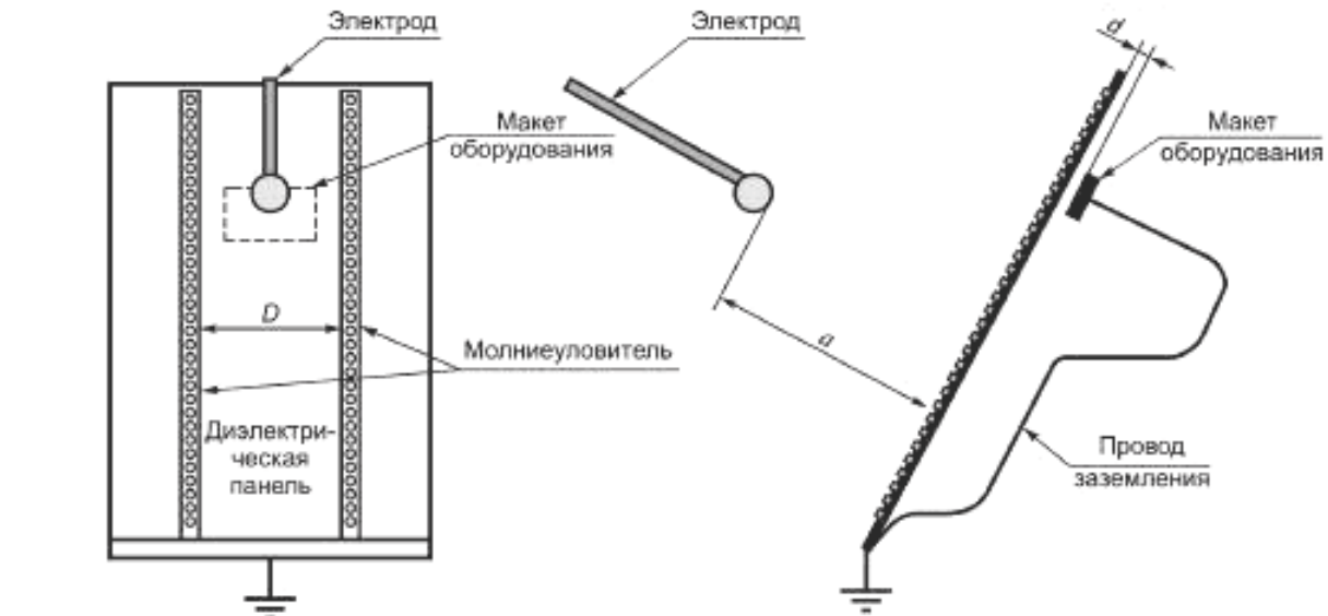
Рисунок D.5 — Схема расположения локального защитного устройства (например, молниеуловителя) — Схема В для оценочных испытаний
