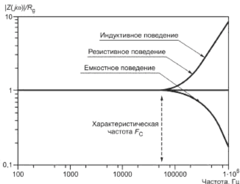
Рисунок 1.2 — Зависимость частоты от полного сопротивления заземления
