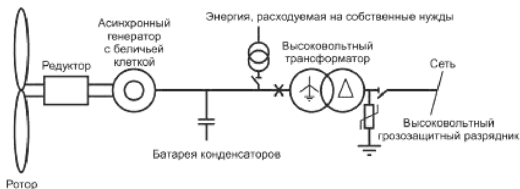
Рисунок 4а — асинхронный генератор с беличьей клеткой
