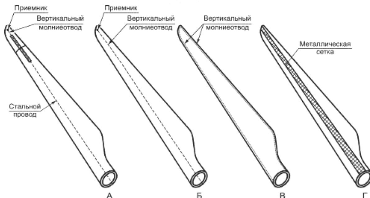
Рисунок С.2 — Принципы молниезащиты для лопастей больших ВЭУ
