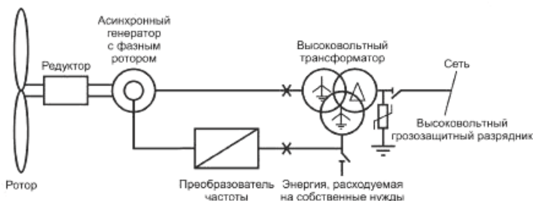
Рисунок 4б — асинхронный генератор с фазным ротором
