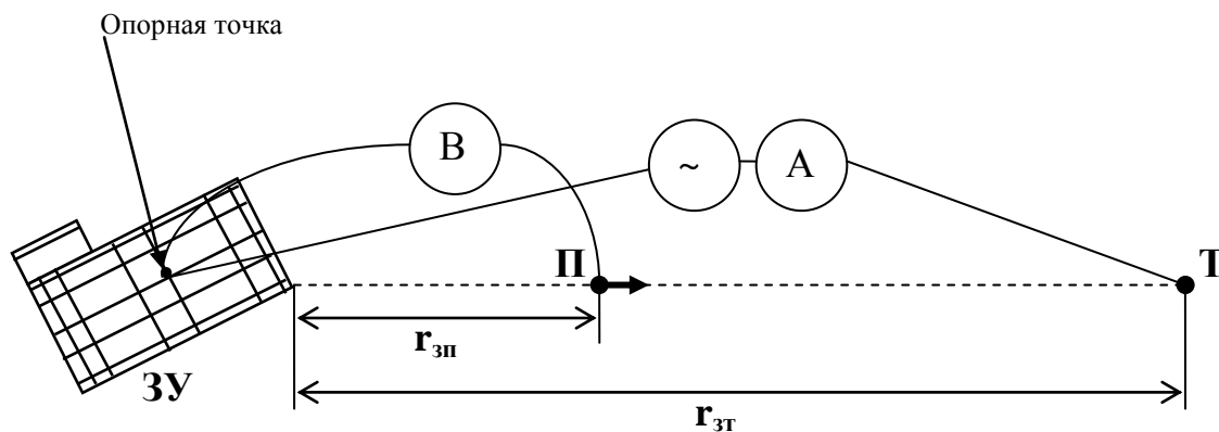
П – потенциальный электрод, Т – токовый электрод Рис. 5. Схема измерения сопротивления заземляющего устройства
